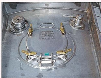
② 安全弁および ③ 通気口
